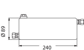
Охладитель импульса давления V1
