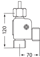
Соединительная деталь KF2, KF3
